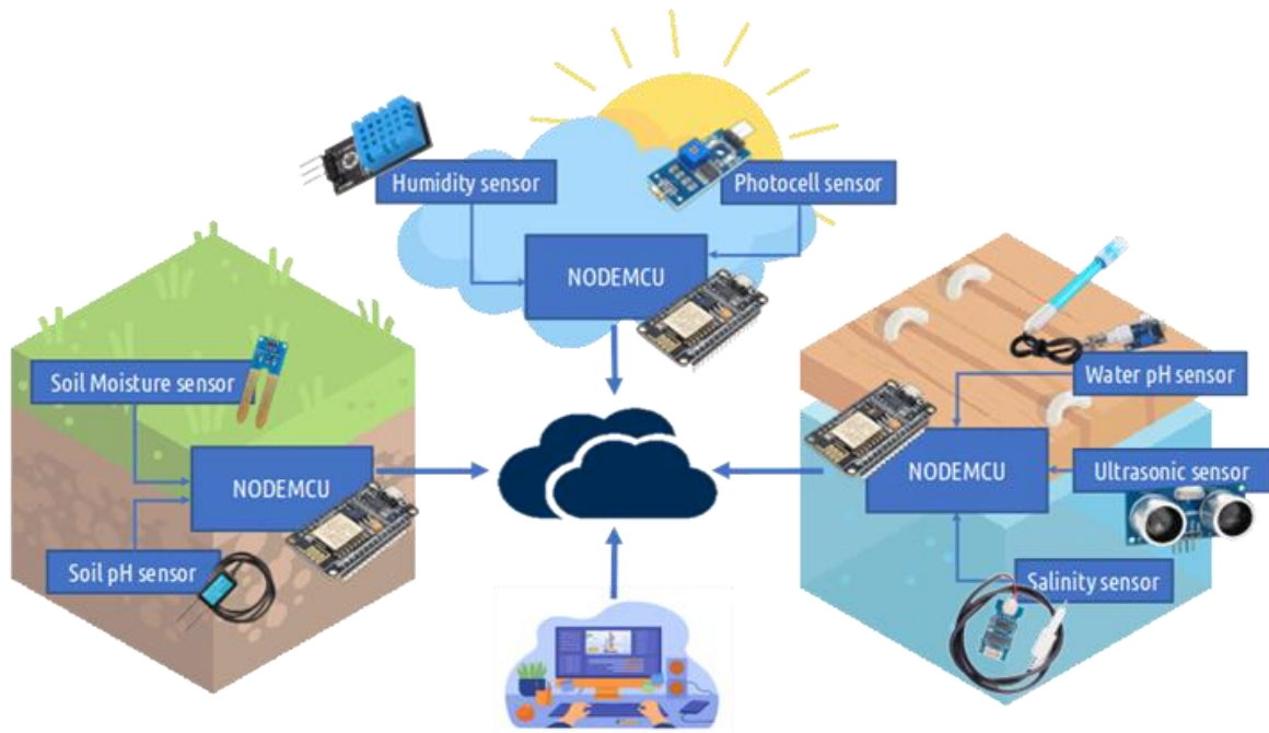
Gambar 1. Rancangan Alat
